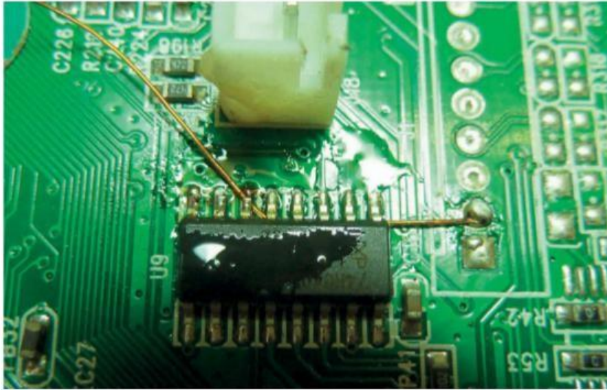
Figure 3-5. Utilisation de fil émaillé
