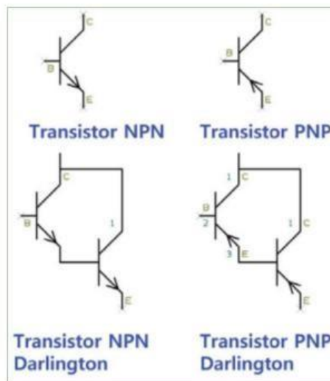
Figure 9-33. Symboles des transistors bipolaires
