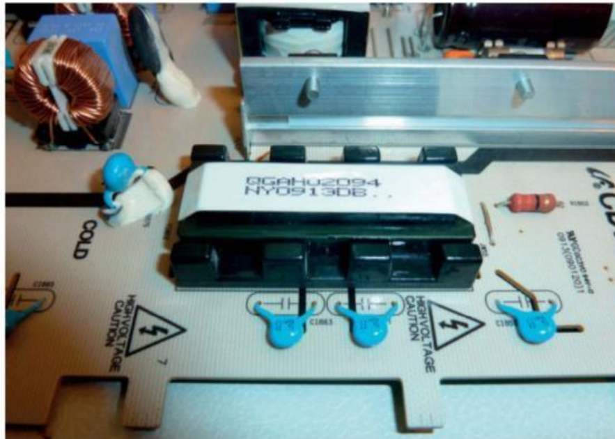
Figure 9-19. Transformateur d'un circuit inverter pour téléviseur LCD
