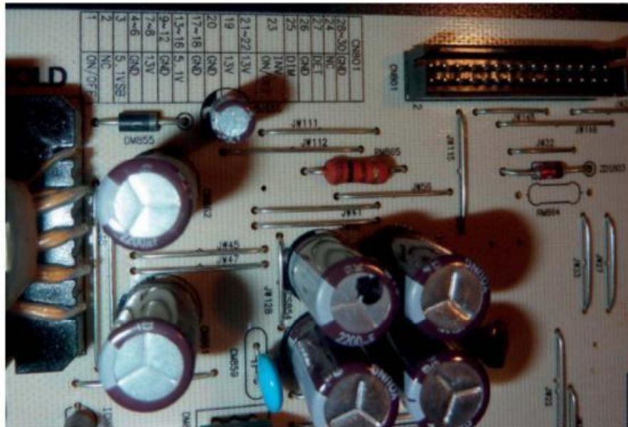
Figure 4-14. Sérigraphie du brochage du connecteur d'une alimentation
