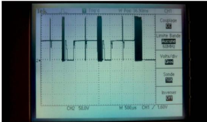
Figure 5-29. Sous-trames de signaux Z-sustain
