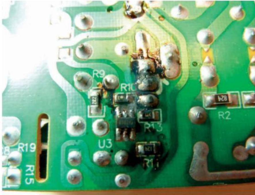
Figure 3-2. Contrôle visuel d'un circuit imprimé d'alimentation
