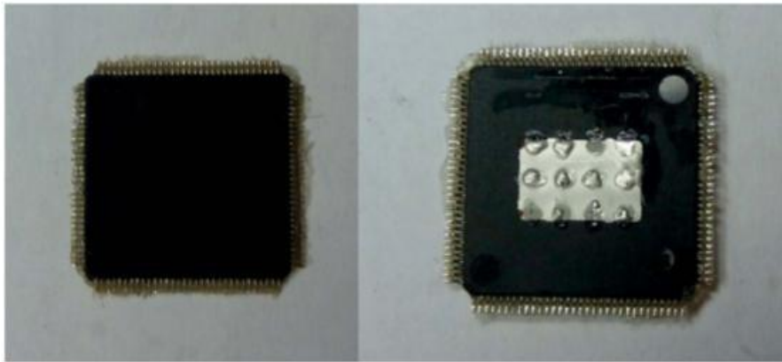
Figure 5-23. Circuit RZA20292BFT avec sa surface de refroidissement sous le boîtier
