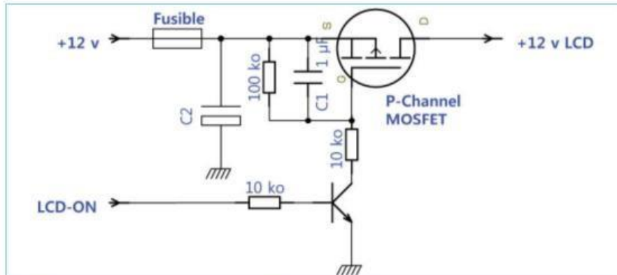
Figure 4-36. Circuit de coupure d'alimentation d'une dalle LCD
