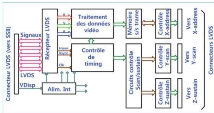
Figure 5-11. Synoptique d'une carte de contrôle logique de dalle plasma
