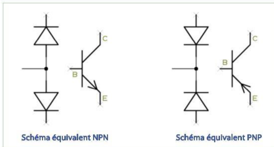
Figure 10-7. Schémas équivalents simplifiés d'un transistor
