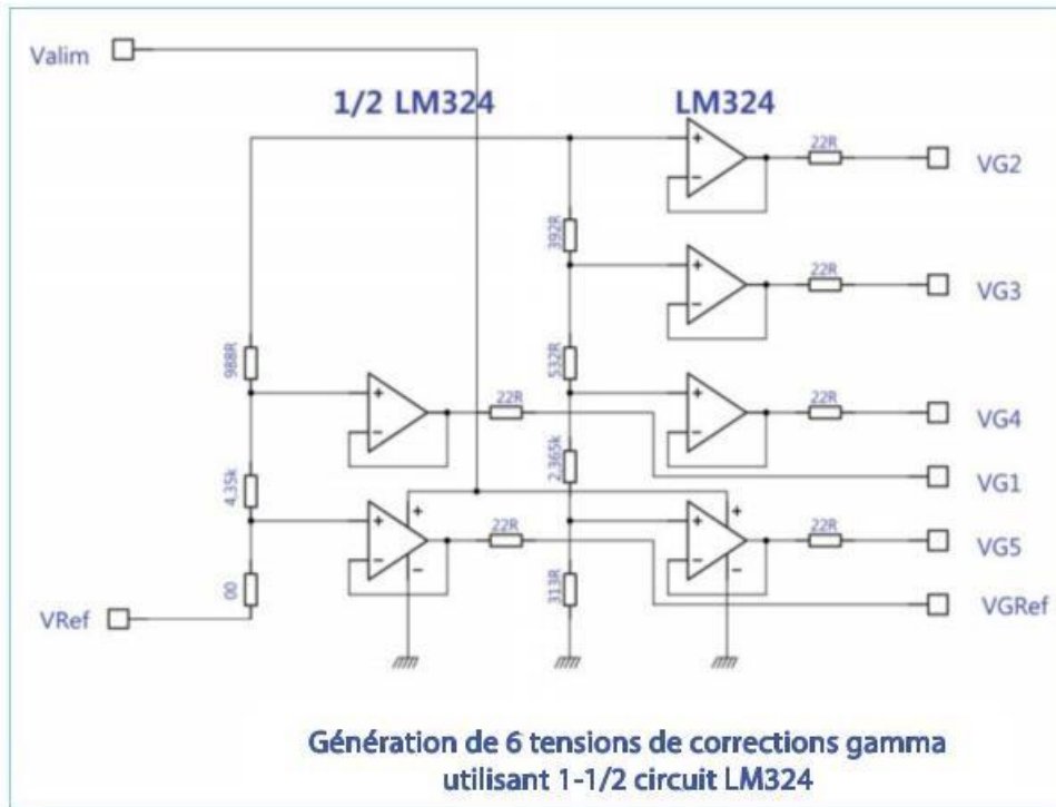
Figure 4-42. Exemple de circuit générateur de tensions de corrections gamma
