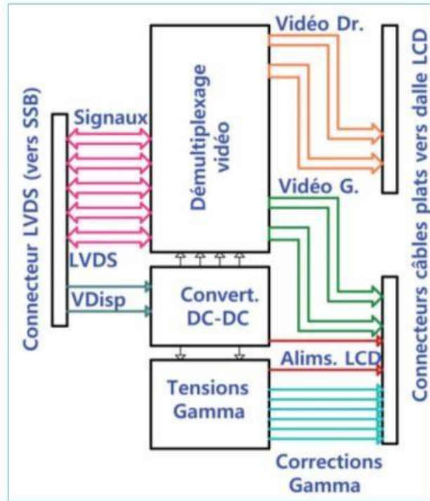
Figure 4-40. Synoptique simplifié d'une carte T-Con
