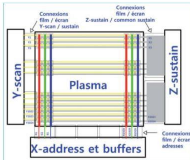
Figure 5-1. Synoptique d'un écran plasma
