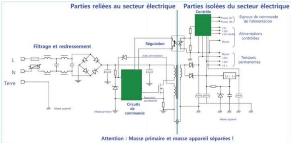
Figure 8-4. Synoptique d'une alimentation à découpage simple
