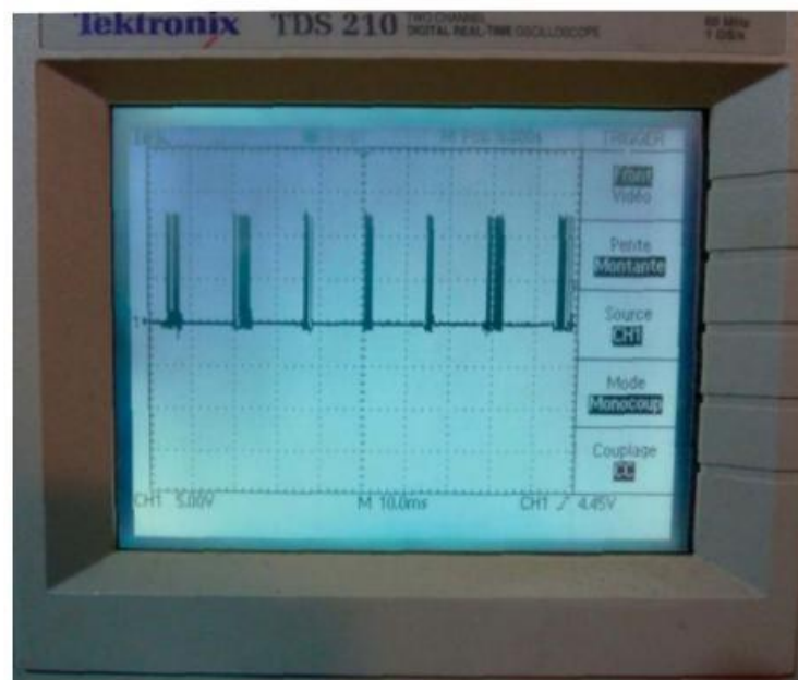
Figure 8-6. Trains d'impulsions sur une alimentation en court-circuit
