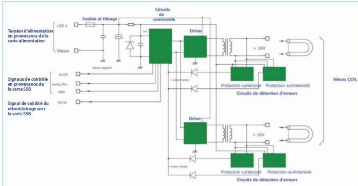
Figure 4-18. Synoptique d'un inverter séparé des circuits d'alimentation
