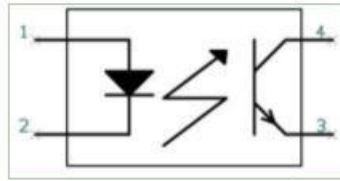
Figure 10-9. Symbole d'un optocoupleur
