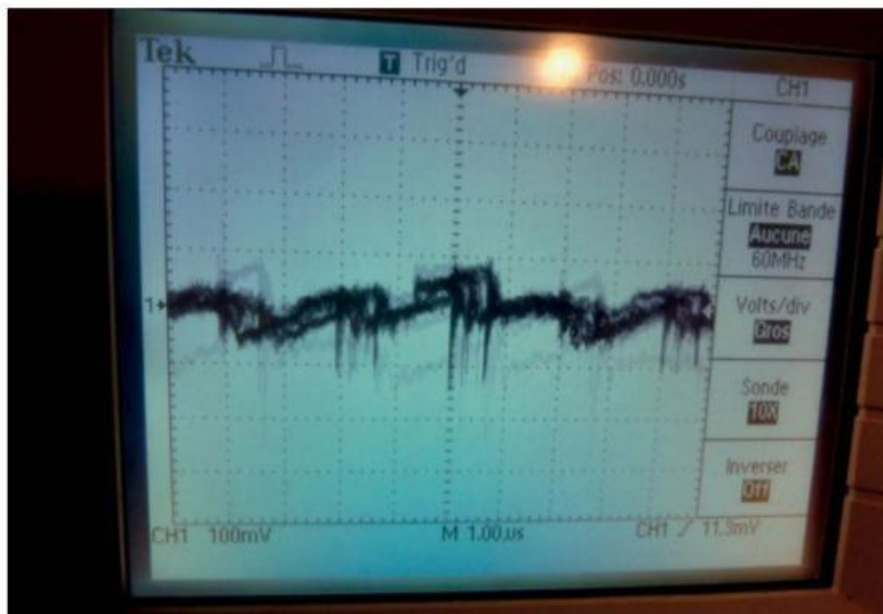
Figure 6-11. Bruit au niveau d'une ligne d'alimentation
