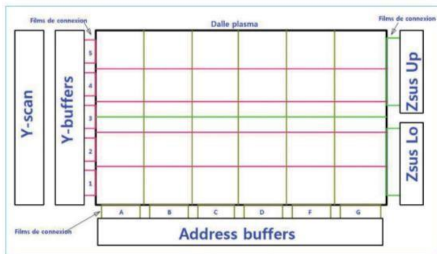
Figure 5-7. Localisation des zones d'un écran plasma
