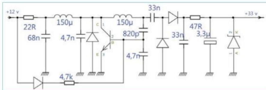
Figure 4-30. Circuits DC/DC éleveur à découpage utilisant un circuit auto-oscillant
