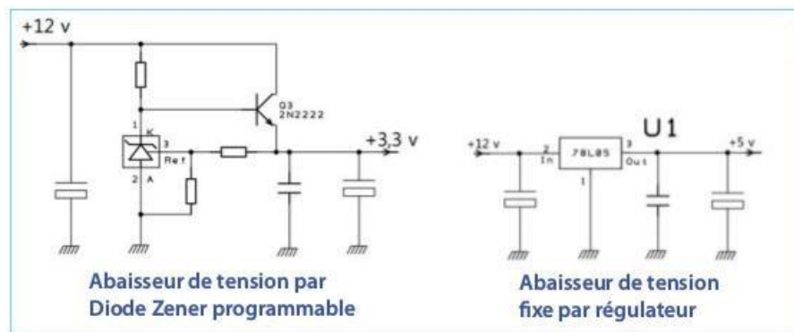
Figure 4-28. Circuits DC/DC abaisseurs simples
