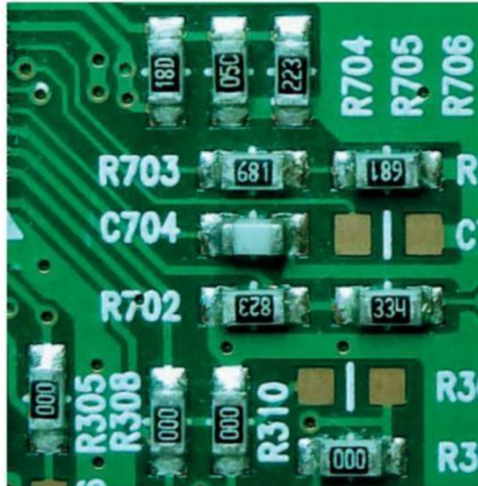
Figure 9-6. Différents marquages de résistances CMS
