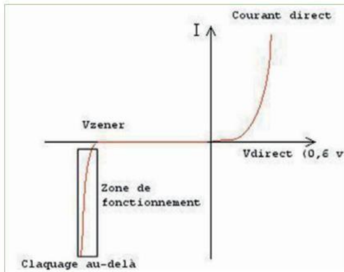
Figure 9-31. Courbe caractéristique d'une diode Zener
