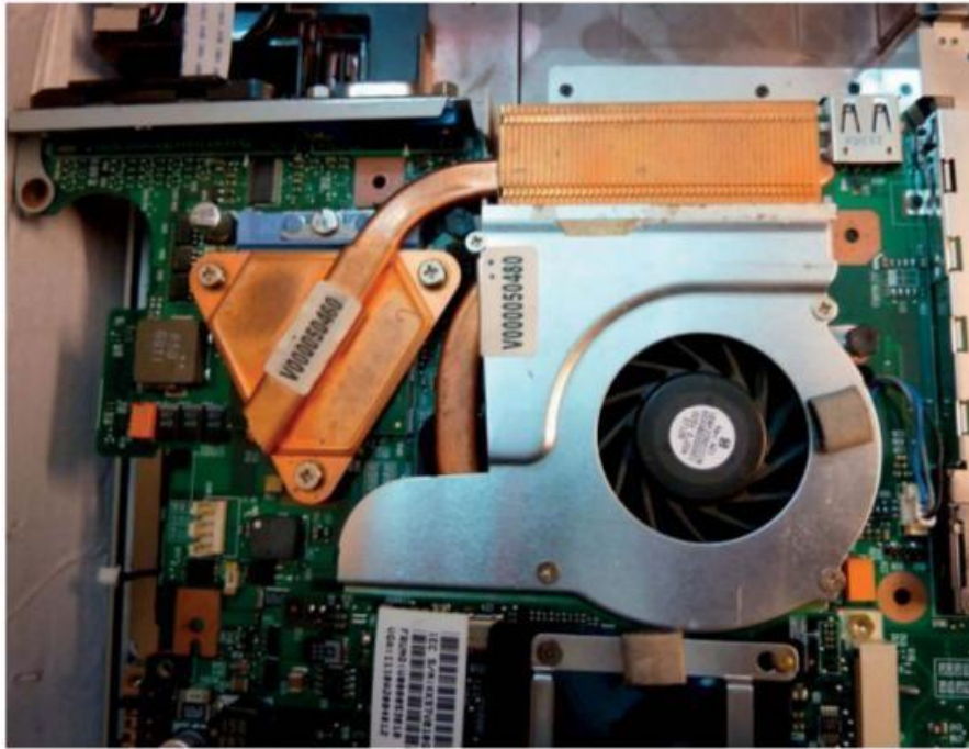
Figure 6-25. Processeur sous la partie triangulaire du refroidisseur
