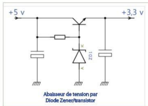
Figure 9-32. Utilisation d'une diode Zener dans un régulateur abaisseur de tension simple
