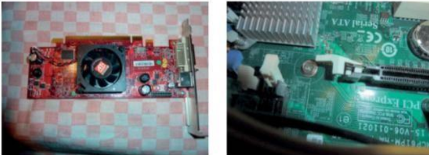
Figure 6-4. Carte vidéo démontée (notez l'ergot et le verrou du connecteur)
