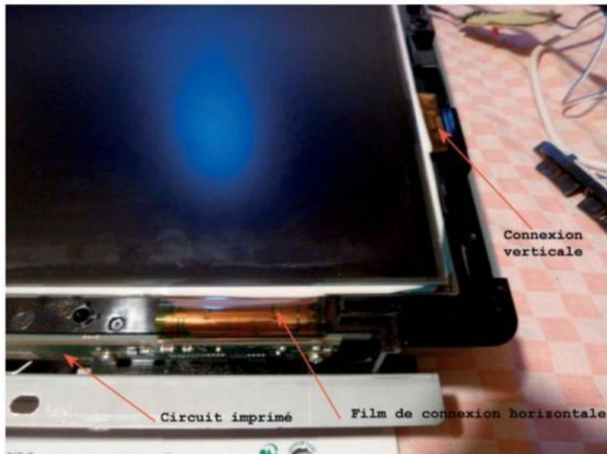
Figure 4-54. Connexions d'un panneau LCD
