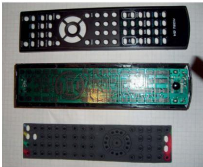
Figure 7-42. Télécommande démontée
