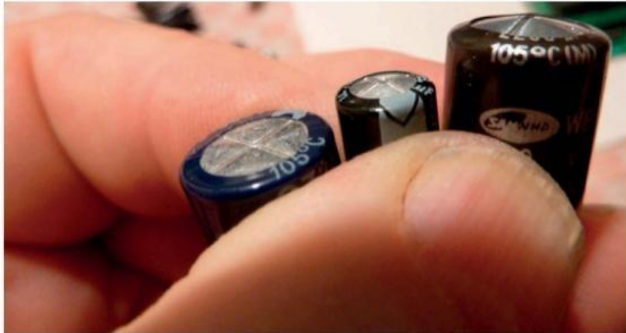
Figure 5-8. Condensateurs électrochimiques : les deux à droite sont anormalement gonflés
