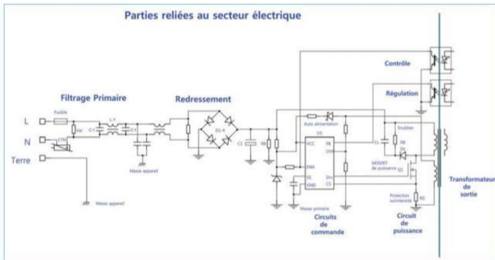
Figure 8-2. Circuit primaire d'une alimentation à découpage
