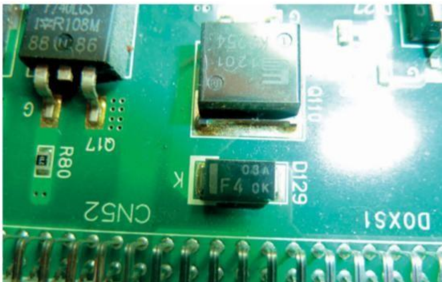
Figure 12-8. Diode CMS marquée F4
