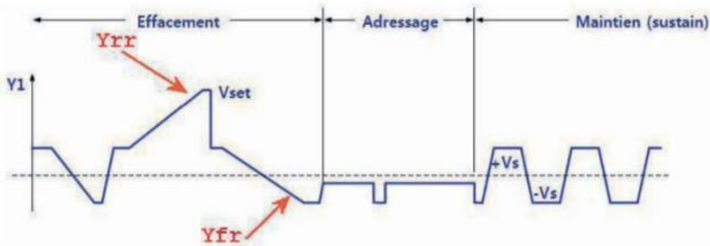
Figure 5-19. Ajustements Yfr et Yrr
