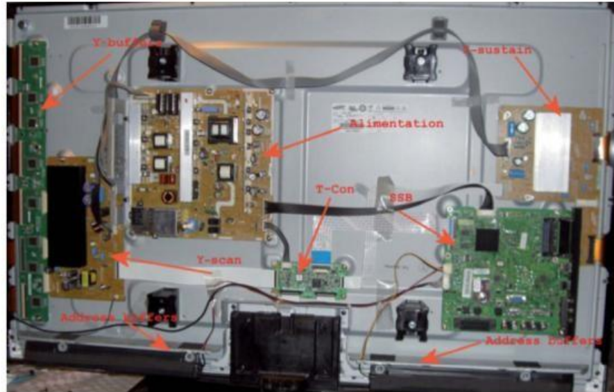
Figure 5-4. Différentes parties d'un téléviseur plasma
