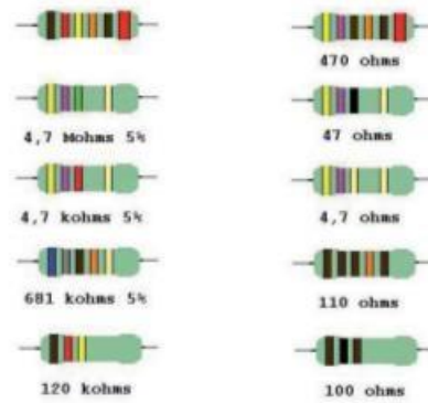
Figure 12-2. Code couleur des résistances : exemples de codifications
