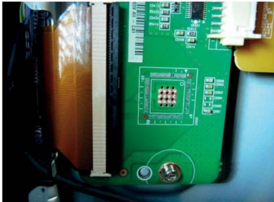
Figure 5-22. Carte Y-buffers après dessoudage du circuit R2A20292BFT
