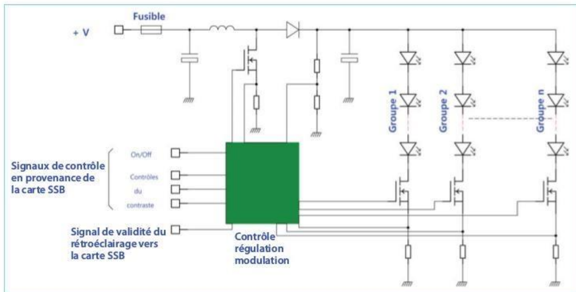
Figure 4-23. Synoptique des circuits de rétroéclairage LED
