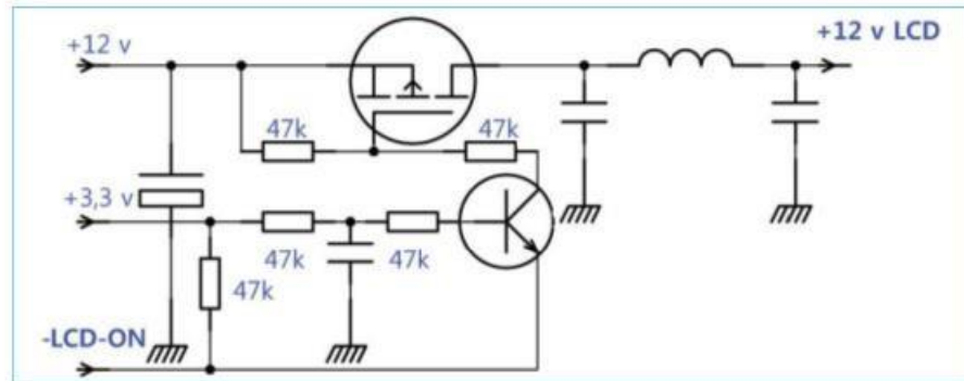
Figure 4-32. Commutation de l'alimentation d'une dalle LCD utilisant un transistor MOSFET P-Channel.
