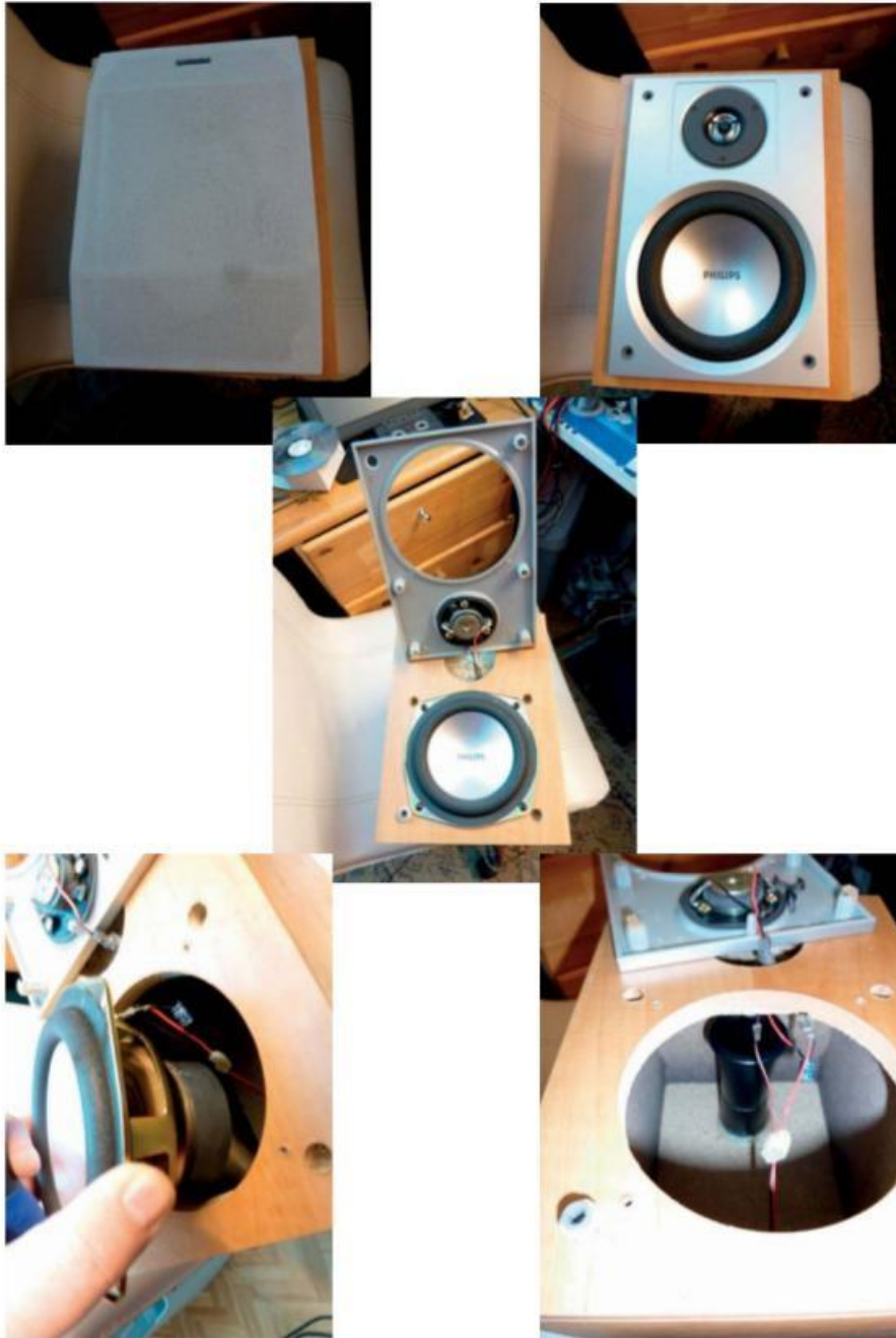
Figure-7-22. Démontage d'une enceinte deux voies
