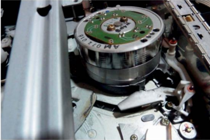
Figure 7-32. Tambour de magnéscope VHS (lecture-enregistrement vidéo)
