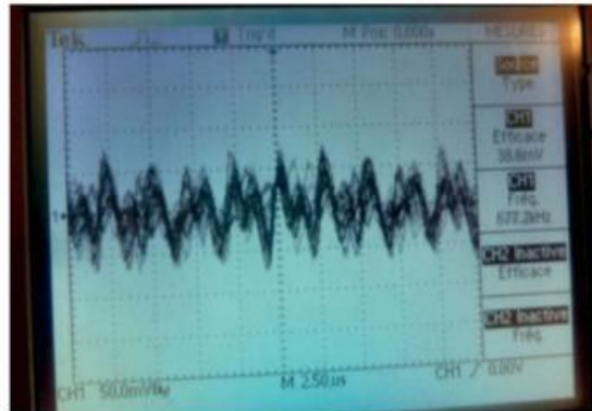
Figure 4-15. Bruit admissible sur une alimentation de 5 volts
