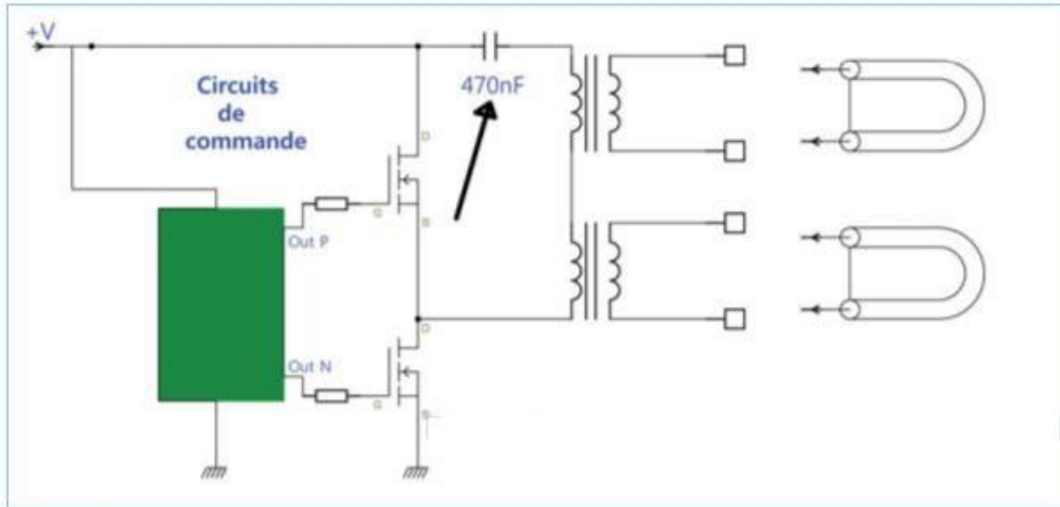
Figure 4-20. Étage de sortie d'inverter montage push-pull avec condensateur de liaison
