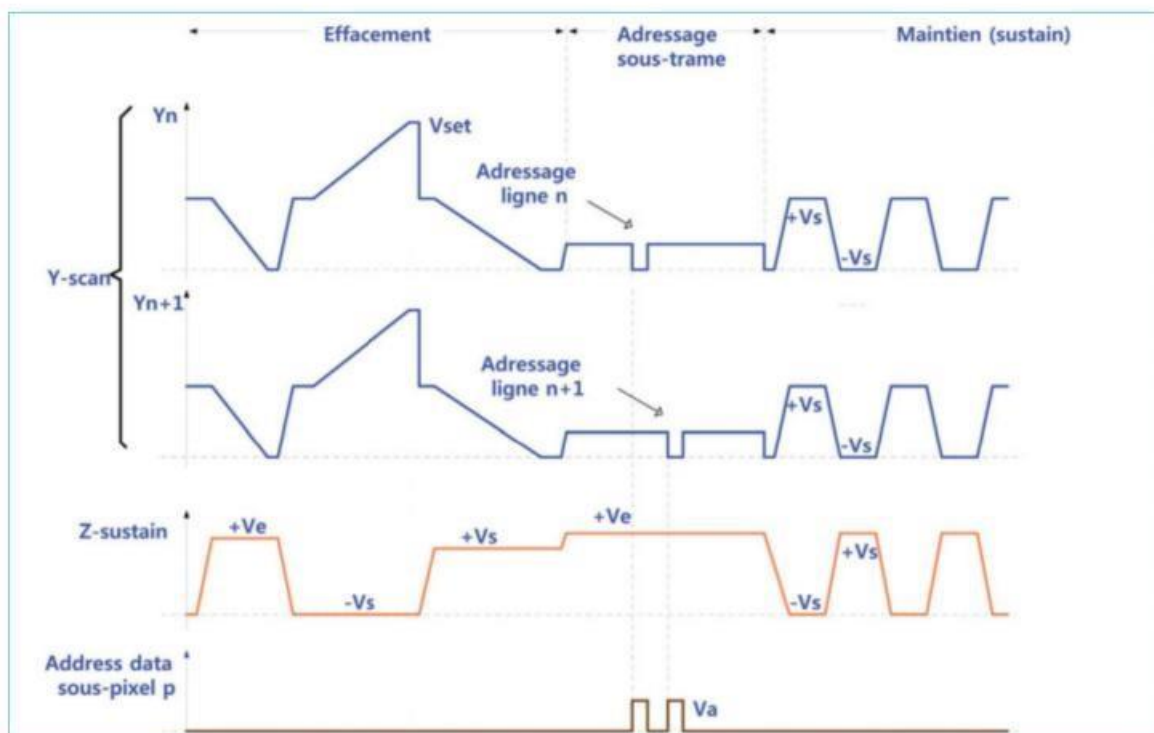
Figure 5-3. Signaux de commande d'affichage de deux sous-pixels superposés de deux lignes consécutives d'un écran plasma
