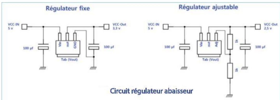
Figure 6-9. Exemple d'utilisation du circuit régulateur
