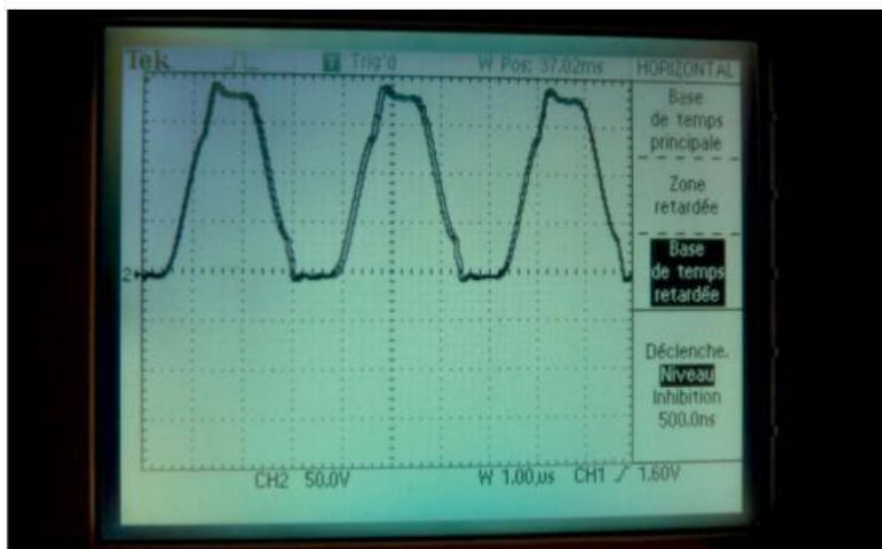
Figure 5-30. Détail des signaux de maintien Z-sustain
