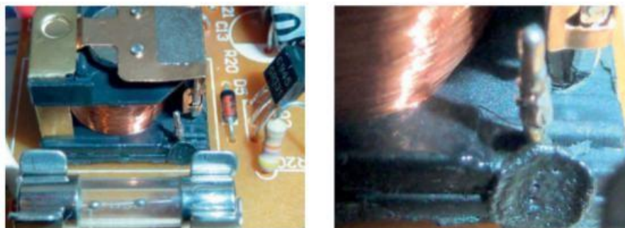
Figure 9-39. Relais avec capot retiré, réparation de la connexion soudée
