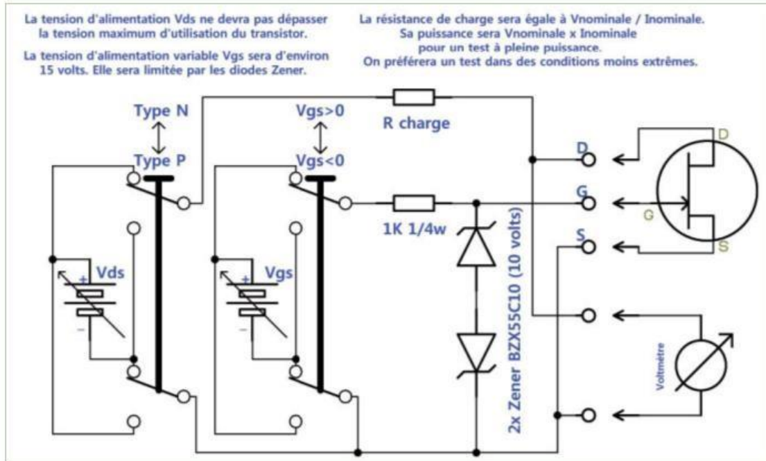
Figure 10-8. Vérification d'un transistor FET
