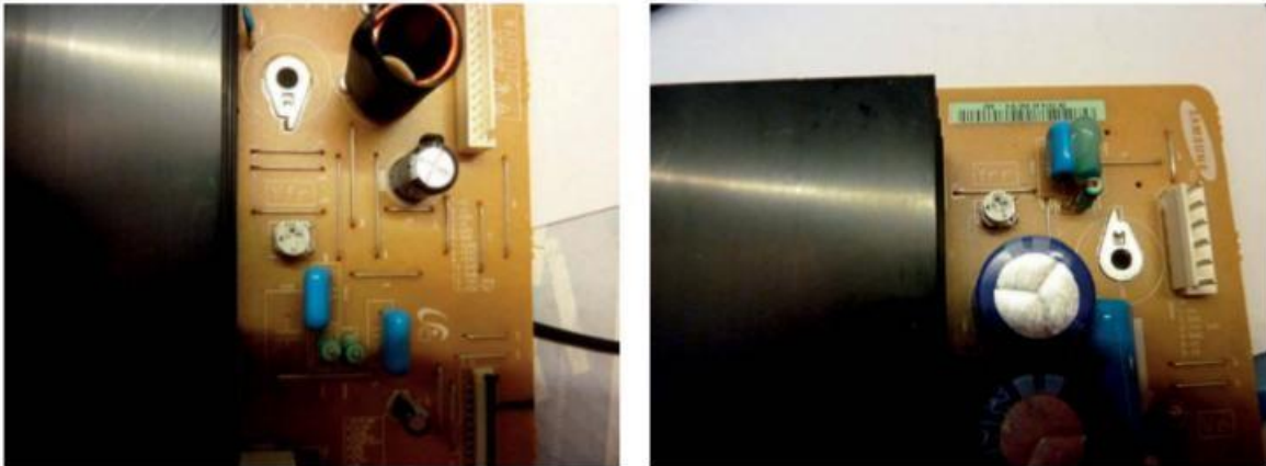
Figure 5-18. Réglage de la forme des signaux d'effacement Y-scan
