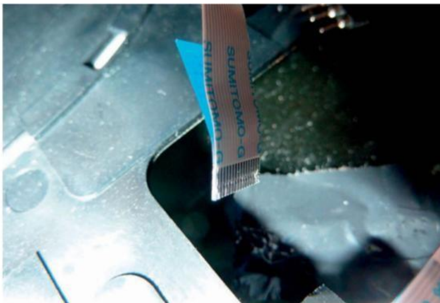
Figure 9-27. Connecteur de câble plat avec languette de manipulation
