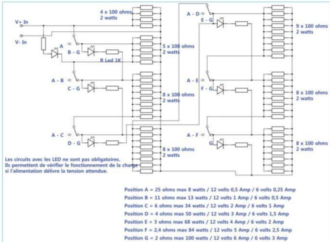
Figure 8-8. Principe d'une charge pour alimentation 3 à 12 V maximum 100 W
