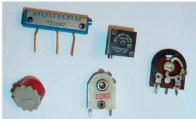
Figure 9-43. Potentiomètres ajustables
