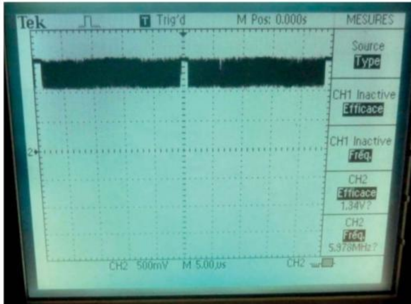
Figure 4-35. Sortie LVDS montrant le signal correspondant à deux lignes vidéo successives (5 µs/div.)
