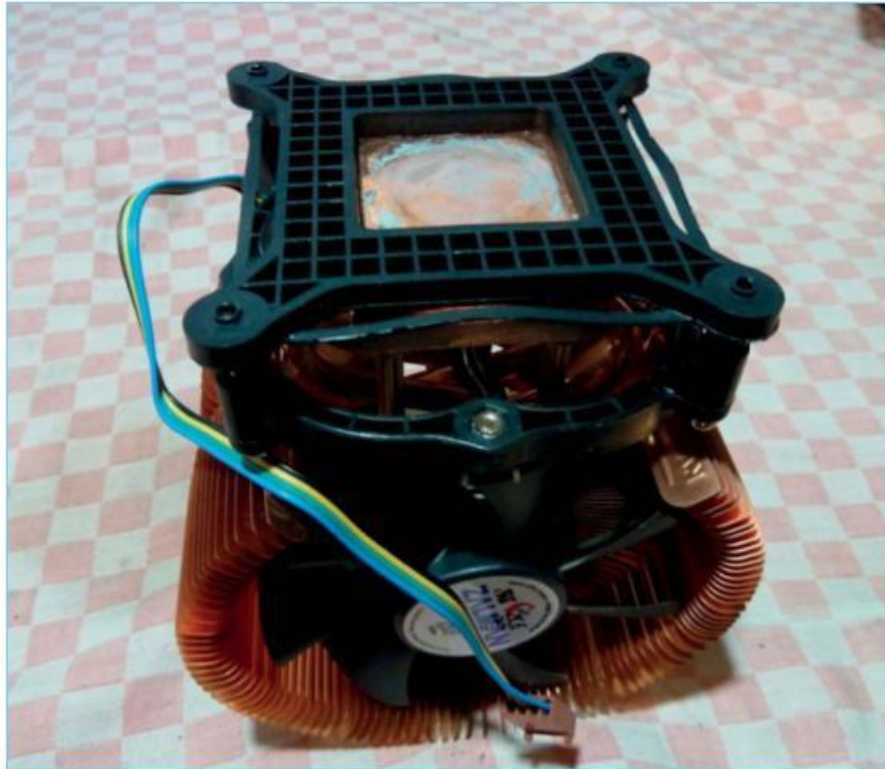
Figure 6-13. Radiateur de microprocesseur récent
