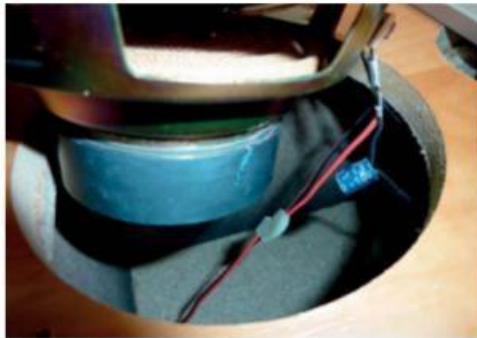
Figure 7-21. Condensateur de connexion vers le tweeter
