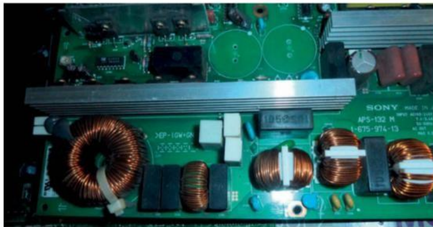
Figure 9-15. Quelques inductances de filtrage du primaire d'une alimentation
