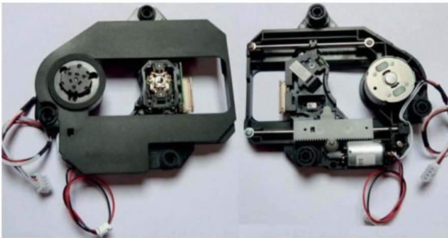
Figure 7-24. Mécanisme complet de lecteur DVD portable
