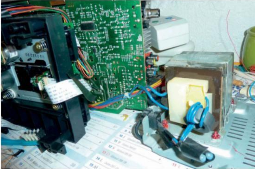
Figure 9-17. Chaîne hi-fi avec transformateur d'alimentation conventionnel (pas à découpage)
