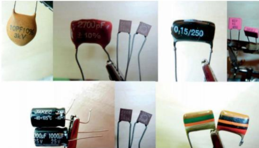
Figure 12-3. Exemples de marquage de condensateurs
