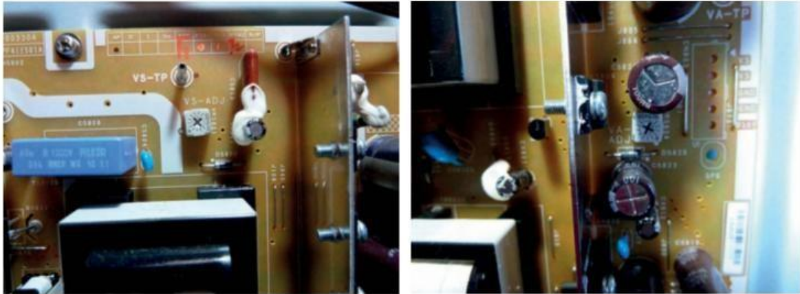
Figure 5-9. Réglages de V_5 et V_6 sur carte d'alimentation
