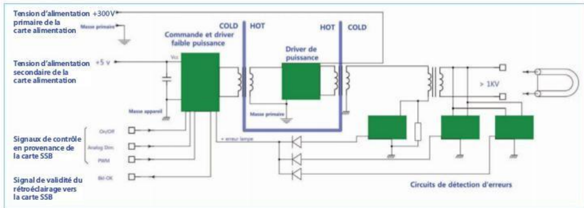
Figure 4-19. Synoptique d'un inverter dans carte alimentation
