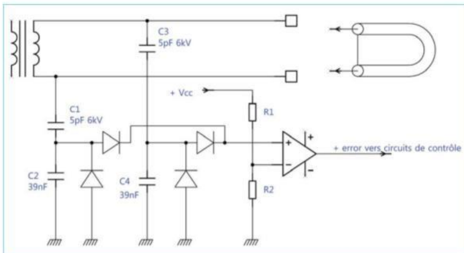
Figure 4-22. Protection surintensité, fuites de tension et déséquilibre des lampes
