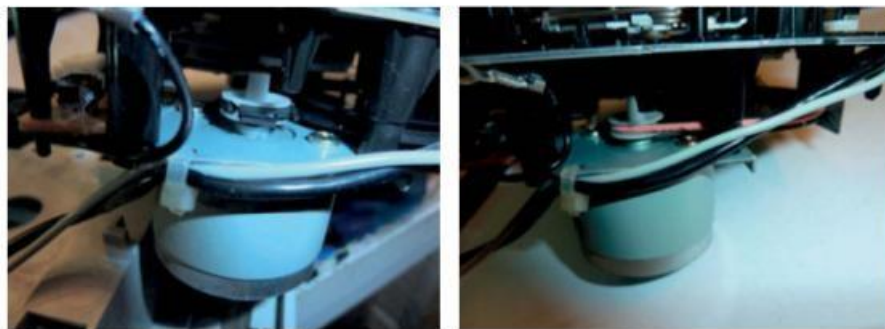
Figure 7-15. Courroie cassée et collée sur sa poulie, remplacée à droite
