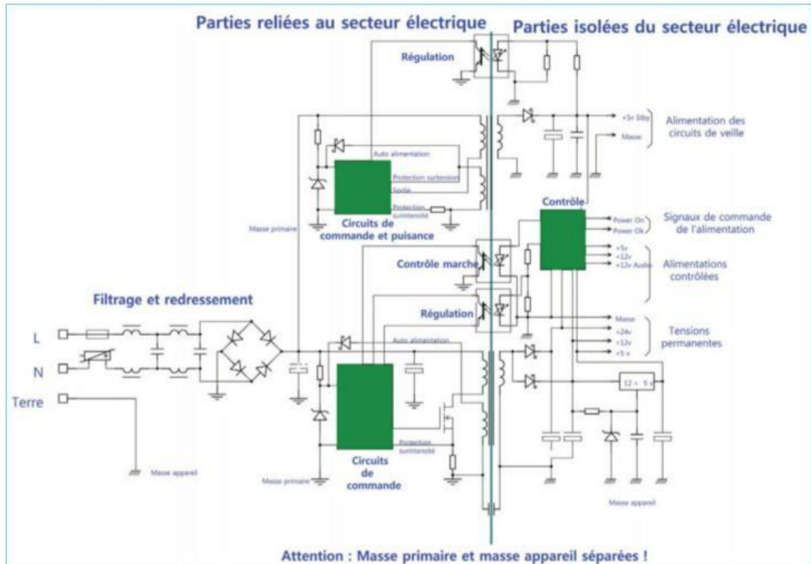
Figure 8-5. Synoptique d'une alimentation à économie d'énergie
