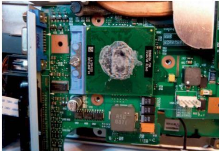
Figure 6-32. Vieillesse de la pâte thermique d'un microprocesseur
