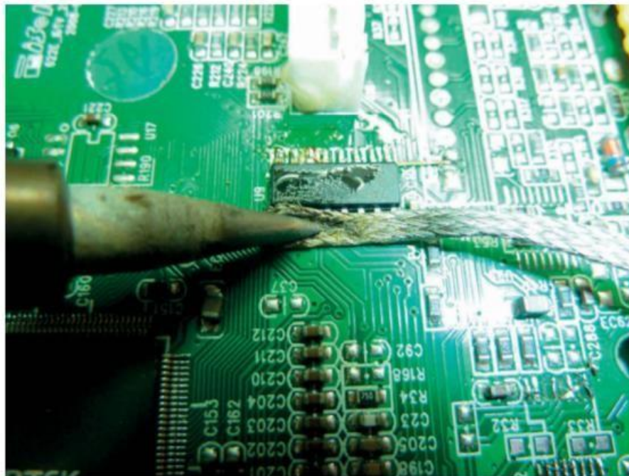
Figure 3-4. Utilisation de tresse à dessouder
