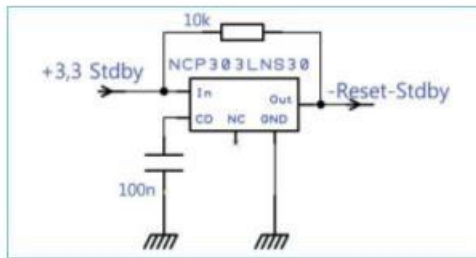
Figure 4-33. Circuit de remise à zéro initiale (reset)
