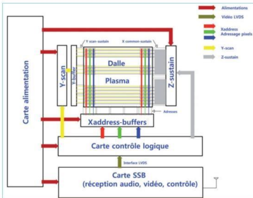
Figure 5-5. Architecture d'un téléviseur plasma
