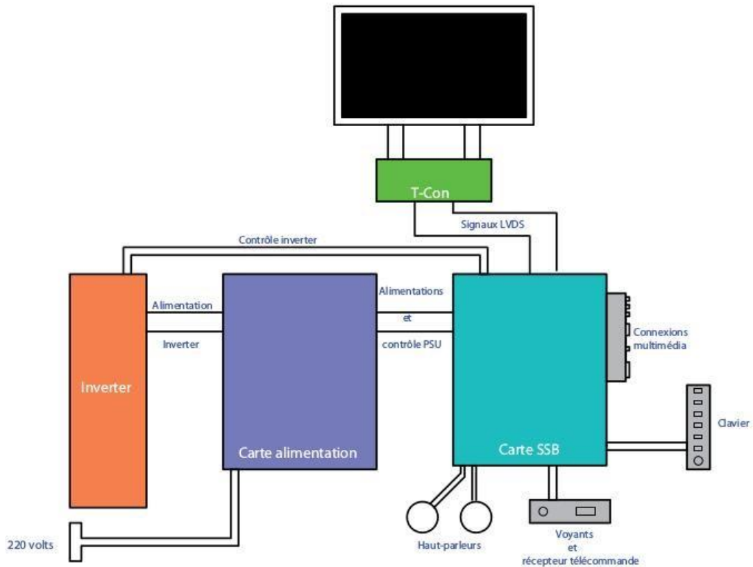
Figure 4-1. Synoptique d'un téléviseur LCD
