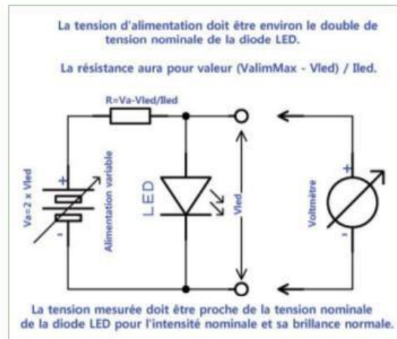
Figure 10-6. Contrôle du fonctionnement d'une diode LED
