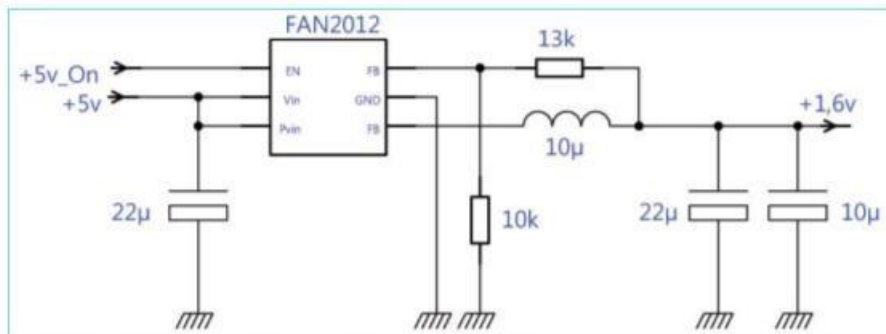
Figure 4-31. Circuits DC/DC abaisseur à découpage utilisant un circuit FAN2012
