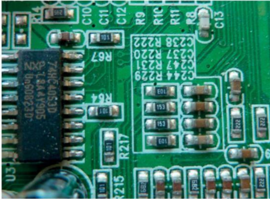
Figure 9-5. Quelques résistances CMS dans leur environnement.
