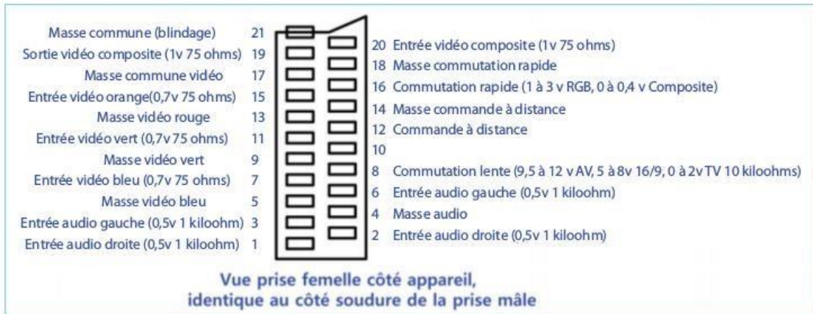
Figure 4-37. Brochage de la prise Péritel
