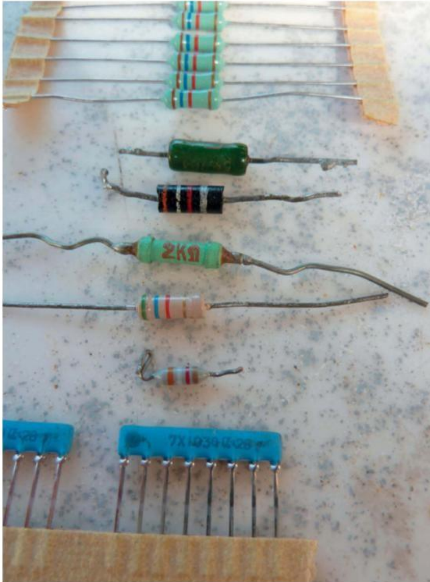
Figure 9-4. Quelques résistances et des réseaux de résistances
