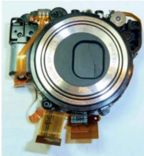
Figure 7-8. Bloc optique d'un appareil photo numérique
