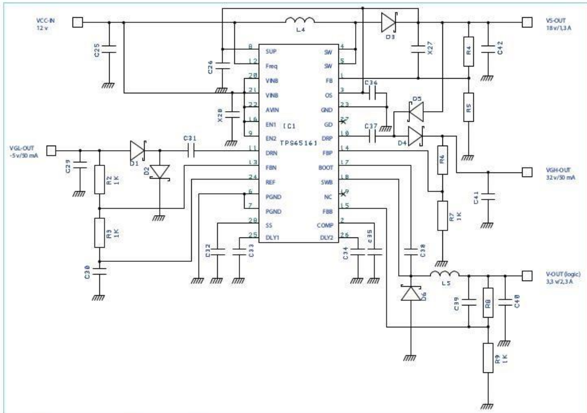
Figure 4-41. Exemple d'alimentations internes d'une carte T-Con
