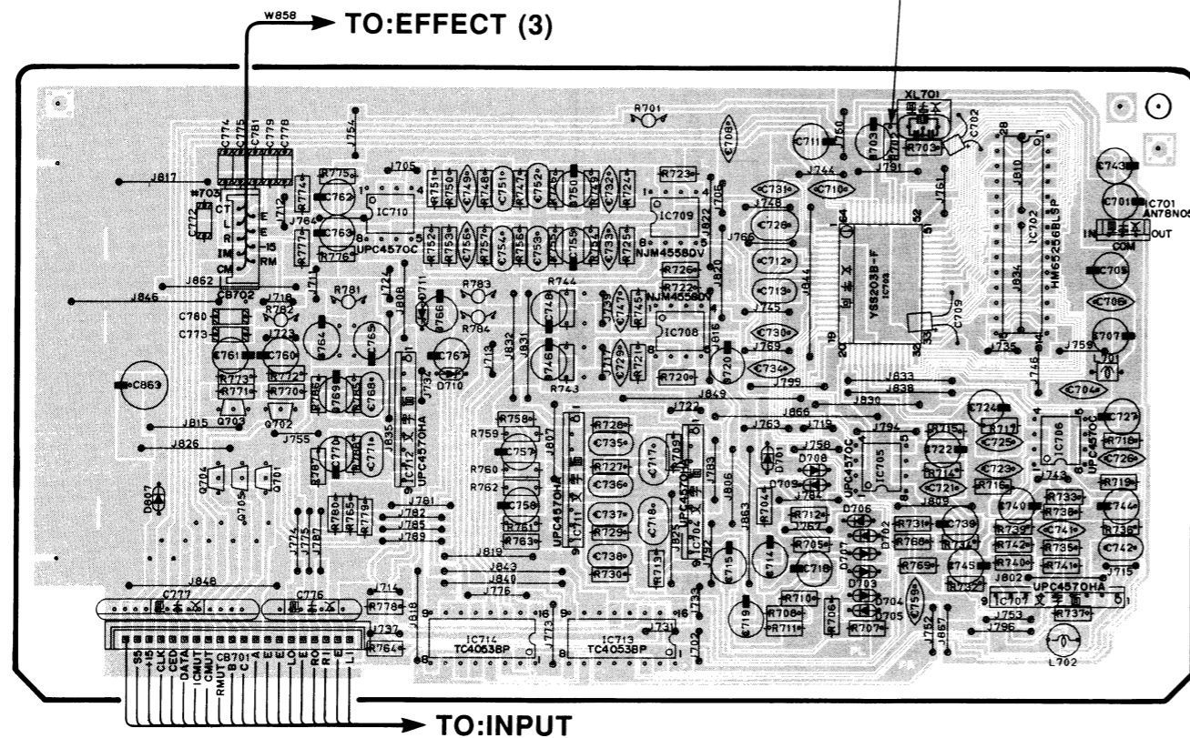
P.C.B. EFFECT ( 1 )
