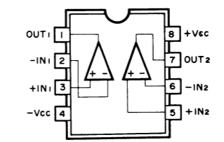
IC705, 706, 710 : \mu PC4570C IC708, 709 : NJM4558DV Dual OP-Amp
