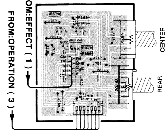
P.C.B. EFFECT ( 3 )
