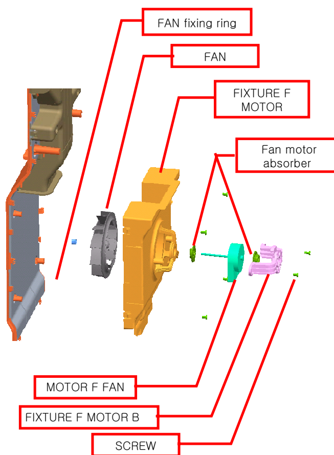
Disassemble drawing for fan & fan motor
