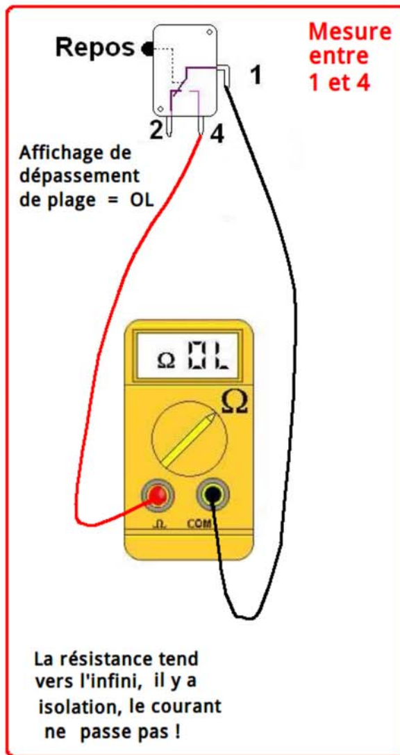
Mesure du contact (1,4) au repos, il y a isolation.
