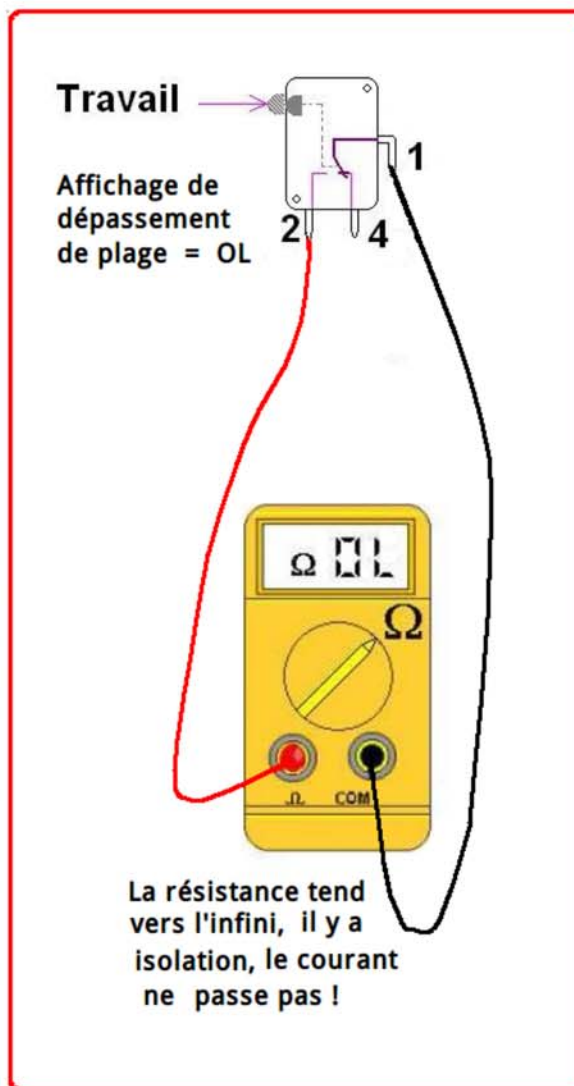
Mesure du contact (1,2) au travail, il y a isolation.
