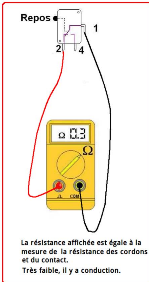
Mesure du contact (1,2) au repos, il y a conduction.
