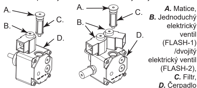
Obrázek 11 - Pumpa hořáku
