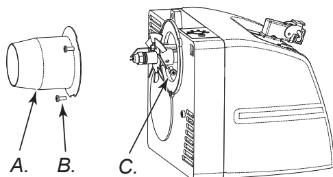
Figura 12 - Smontaggio canotto-bruciatore
