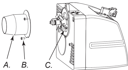
Figur 12 - Demontering rør-brenner
