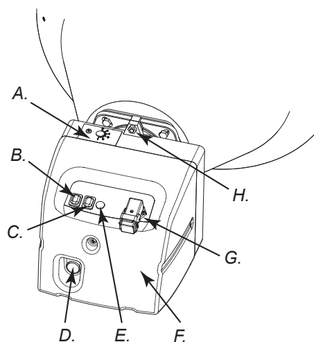
Рисунок 5 - Устройства, контролирующие работу нагревателя
