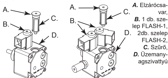
11 Ábra - Üzemanyagszivattyú
