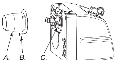
Abbildung 12 - Demontage rohr und brenner
