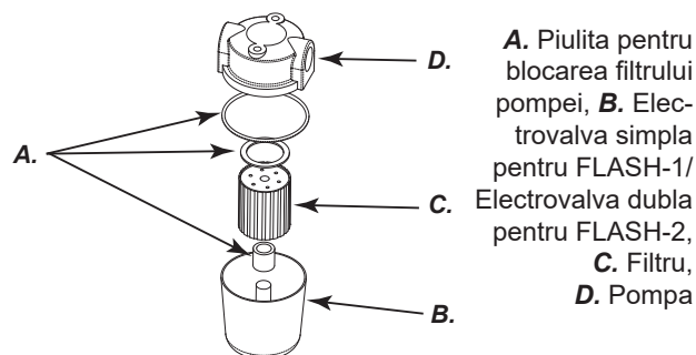
Figura 10 - Filtrul încălzitorului
