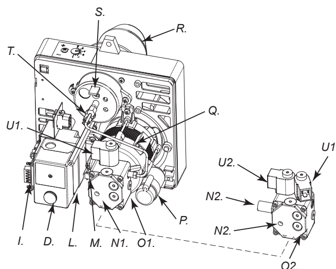
Abbildung 6 - Brennerkomponenten
