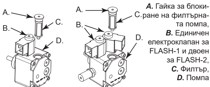
Фигура 11 - Филтър на отоплителя
