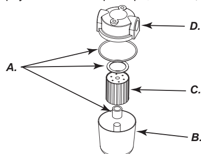
Рисунок 10 - Фильтр нагревателя
