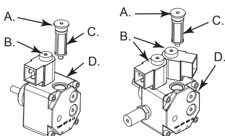
Figura 11 - Bomba del quemador
