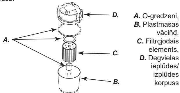
10 Zīmējums - Filtrs
