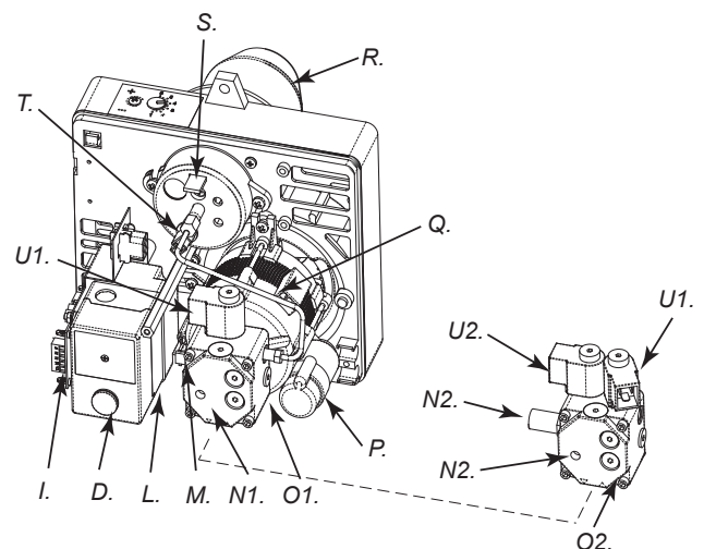
6 Zîmçjums - Degd'a elementi
