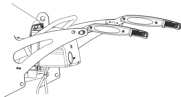
Joonis 9 - Soojendi käepidemed transpordiasendis
