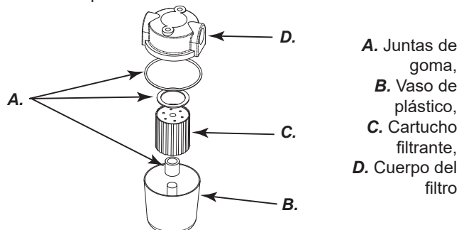
Figura 10 - Filtro de gasóleo
