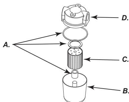
Kuva 10 - Suodatin
