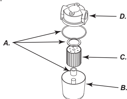
Joonis 10 - Soojendi filter
