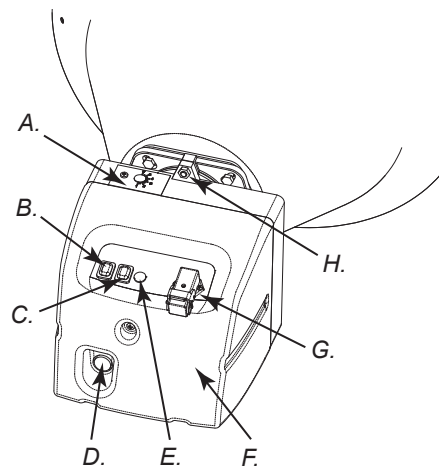
5 Zîmçjums - Vadîbas pogas
