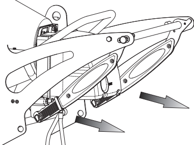
Figura 8 - Posizione maniglie chiuse
