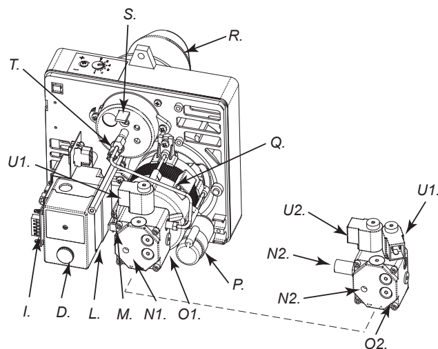
Figur 6 - Brennerens komponenter
