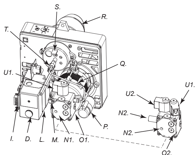
Figur 6 - Brænder og bestanddeile
