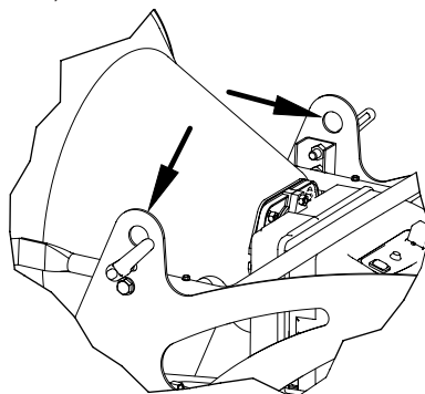
Joonis 7 - Tõstekõrv transportiasendis
