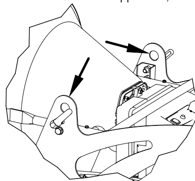
Figur 7 - Festeboltene
