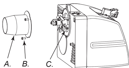
Figura 12 - Demontarea arzătorului
