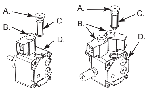
Kuva 11 - Polttimen pumppu
