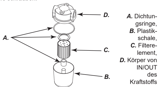
Abbildung 10 - Filter
