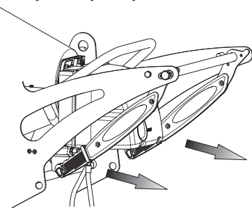
8 Ábra - Hőszugárzó, mozgatókarok zárt pozícióban
