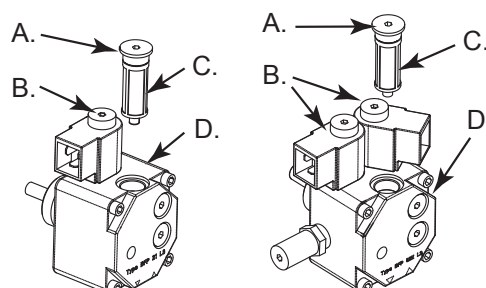
Joonis 11 - Põleti demontaaž
