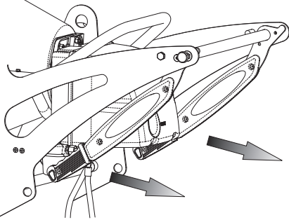
Figura 8 - Mânerele încălzitorului în poziția de așteptare
