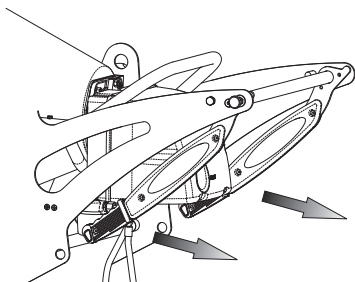
Сурет 8 - Фиксациялау қалпындағы ұстағыштар, жылытқыш
