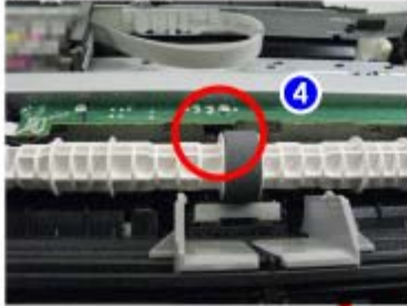
4. PE sensor
