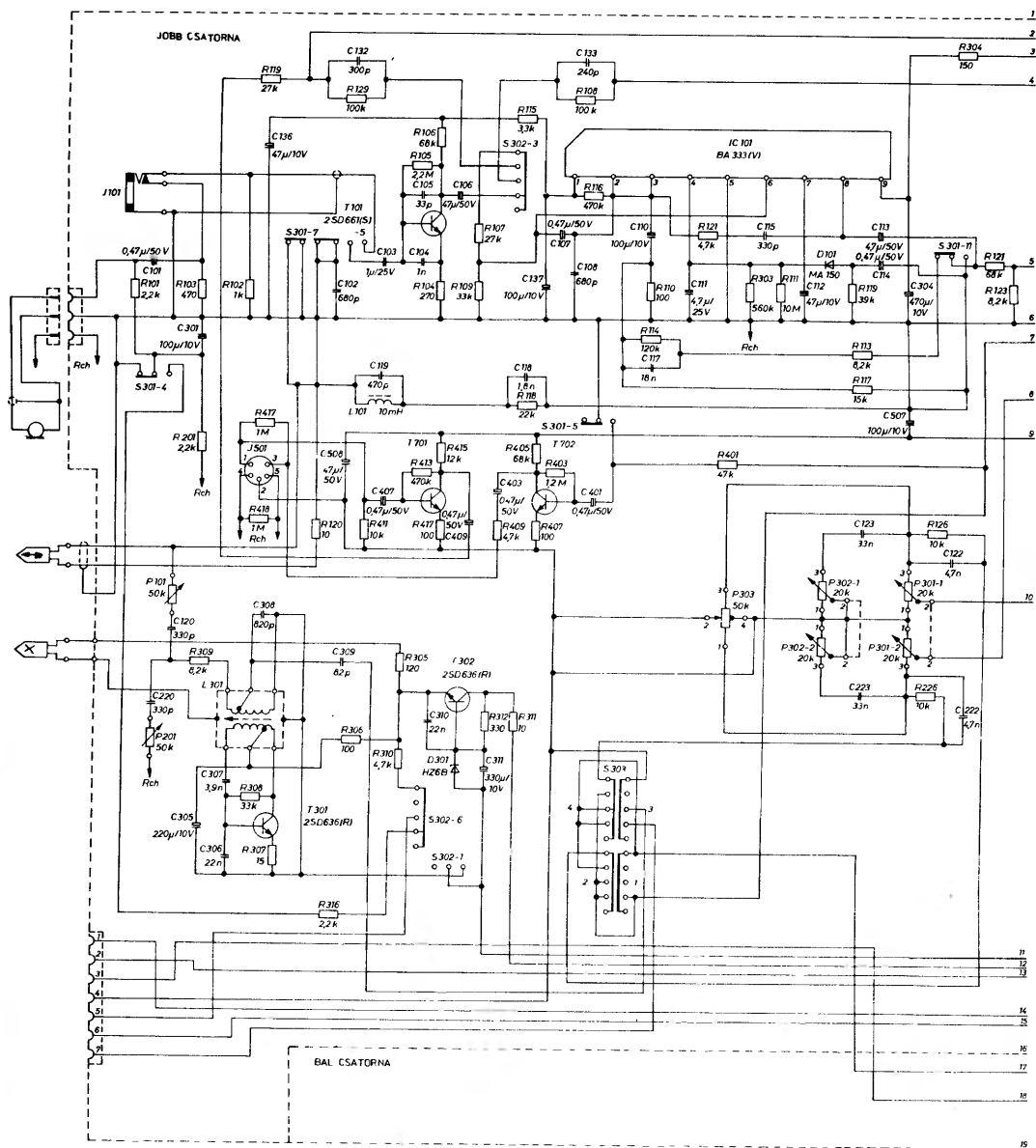
146. ábra A JVC RC 555 áramköreinek kapcsolási vázlata
